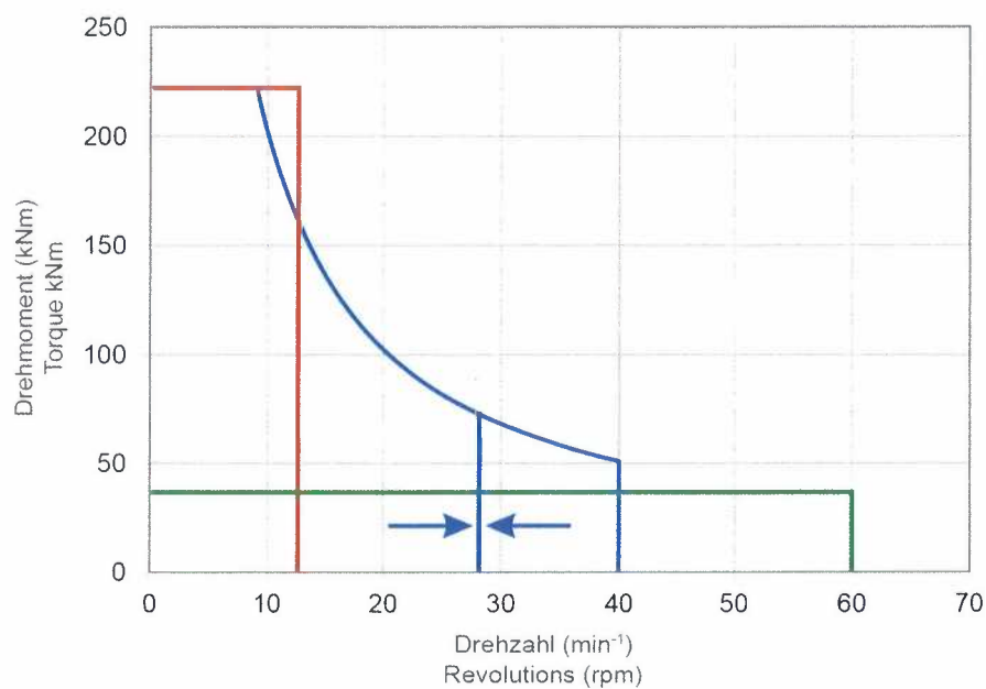
Kellybohrantrieb BT 220 / Rotary Head BT 220
